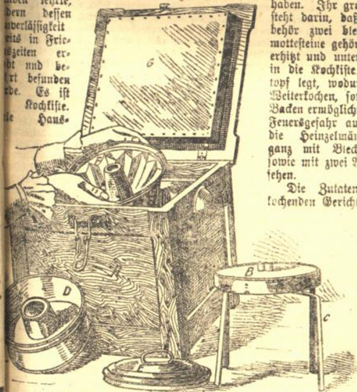
Abbildung 1. Heintzelmannchen-Apparat mit einer Kochkiste. A Holzbox aus feineren Holzern. B Schamotteplatte (Wärmespeicher). C Hohes Backblech. D E Fuhdingsern und Deckel. F Backform. G Schlussschloß, isoliert.
