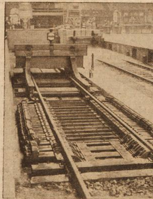
Ein neuer Bremsprellblock mit Schlepplrost auf dem Stettiner Bahnhof in Berlin.
